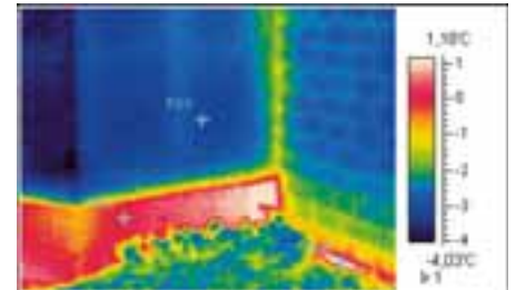
Thermografie: Mit einer Wärmebilddaufnahme wird schnell deutlich, wo die fürs Auge unsichtbaren Schwachstellen eines Gebäudes sind
